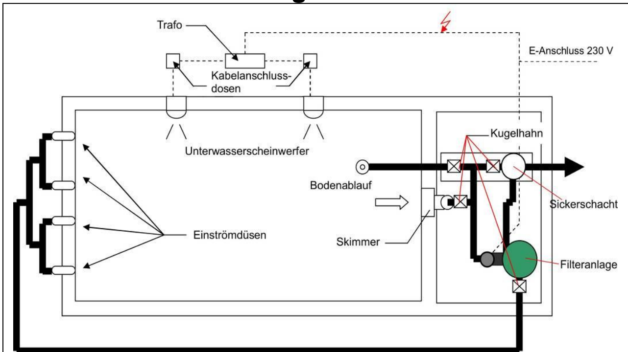
Leitungsschema für Ökopool 8 x 4 m Unterwasserscheinwerfer, Trafo und Kabelanschlussdosen nicht im Set enthalten!
