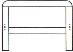
② 25x983x723 - 1
